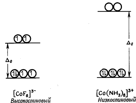
Рис. 12. Относительные величины расщепления кристаллическим полем ( \Delta_0 ) d -орбит высокоспиновых и низкоспиновых октаэдрических комплексов Co(III).
