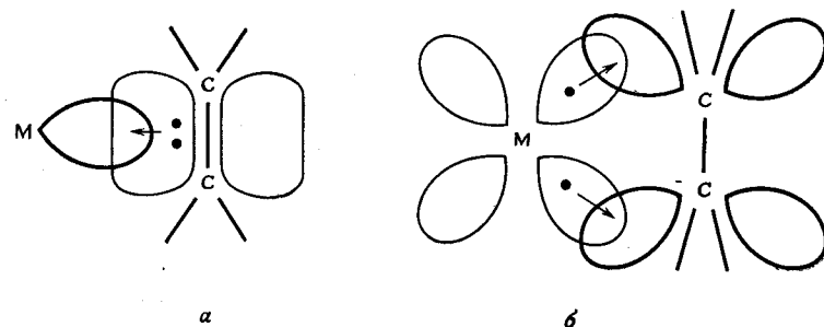
Рис. 29. Изображение связи металл — олефин в комплексах. а — \sigma -связь, образующаяся за счет перекрывания \pi -МО олефина с орбитой металла; б — \pi -связь, образующаяся за счет перекрывания \pi^* -разрыхляющей МО олефина с d -орбитой металла.
