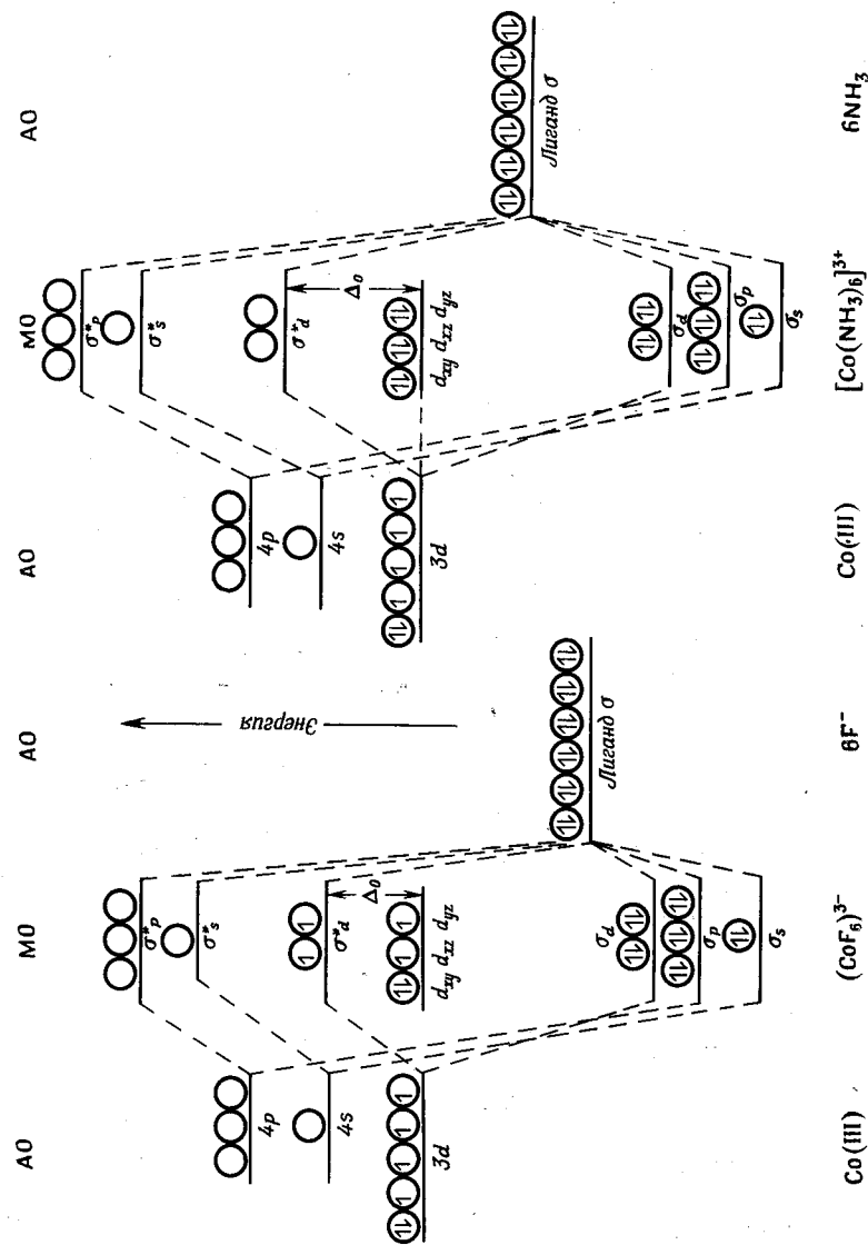
Р и с. 20. Диаграмма уровней энергии МО высокоспинового комплекса [\text{CoF}_6]^{3-} и низкоспинового комплекса [\text{Co}(\text{NH}_3)_6]^{3+} .
