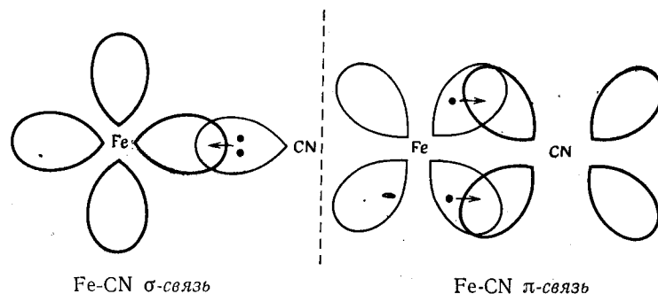
Рис. 21. \sigma - и \pi -Связи в комплексе [\text{Fe}(\text{CN})_6]^{4-} . \pi -Связь образуется за счет использования заполненной d -орбиты иона \text{Fe}^{2+} и пустой разрыхляющей \pi^* -орбиты \text{CN}^- (см. \pi^* на рис. 16).
