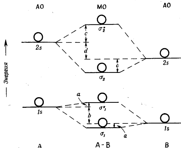
Рис. 19. Диаграмма уровней энергии молекулярных орбит молекулы АВ.
