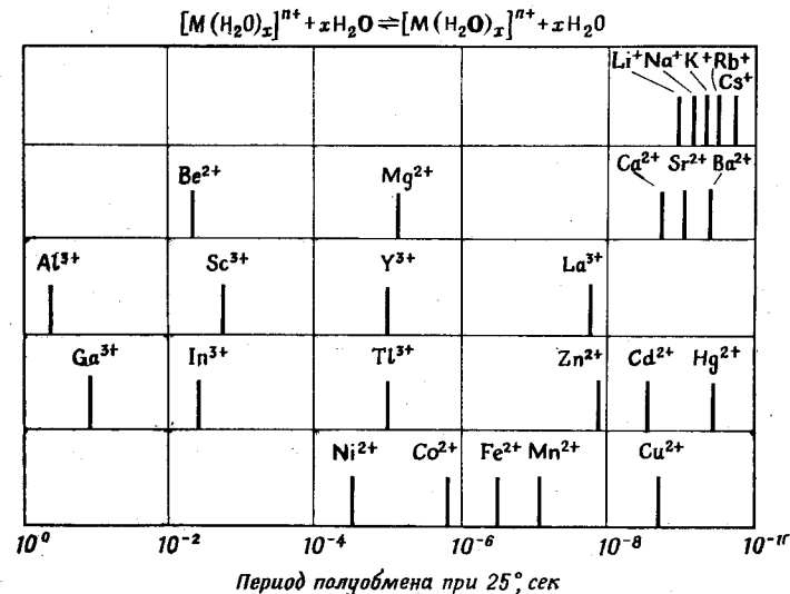
Р и с. 35. Период полуобмена воды для гидратированных ионов металлов. [По данным статьи M. E i g e n, Pure Appl. Chem., 6, 105 (1963).]
