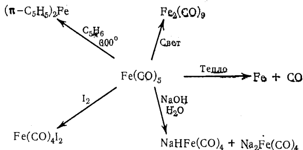
Рис. 28. Реакции с \text{Fe}(\text{CO})_5 , иллюстрирующие химические свойства карбонилы металлов.
