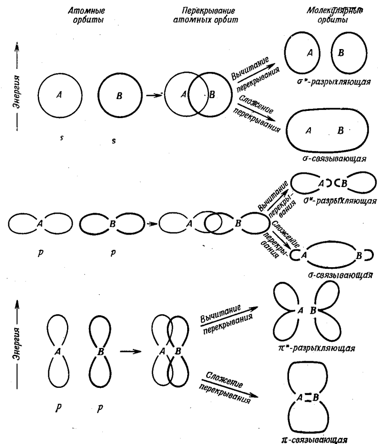
Рис. 16. Образование молекулярных орбит по методу ЛКАО.
