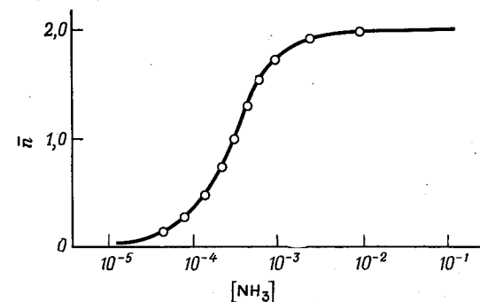
Р и с. 32. Среднее число молекул \text{NH}_3 , связанных с одним ионом \text{Ag}^+ , в зависимости от концентрации свободного аммиака в растворе. Данные приведены для 30^\circ и 2,0M раствора \text{NH}_4\text{NO}_3 .
