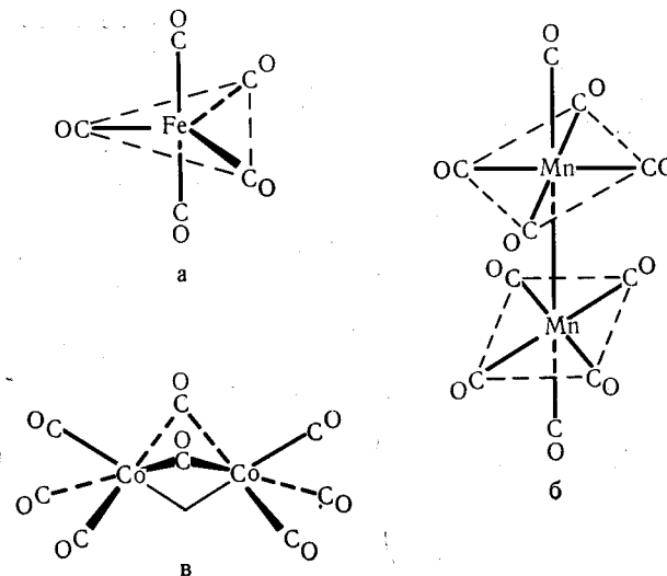
Р и с. 27. Структуры. а — \text{Fe}(\text{CO})_5 , б — \text{Mn}_2(\text{CO})_{10} и в — \text{Co}_2(\text{CO})_8 .
