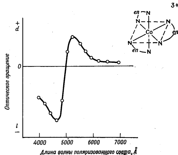
Р и с. 24. Кривые вращательной дисперсии и структуры оптических изомеров [Co(en) 3 ] 3+ .
