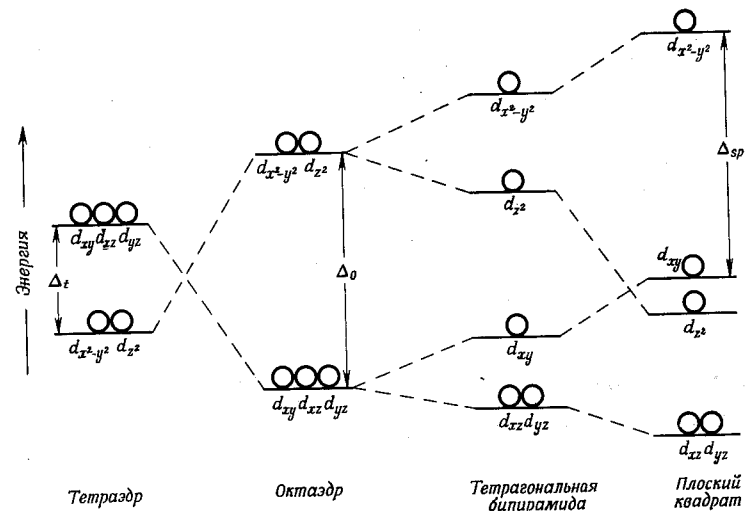
Р и с. 10. Схема расщепления кристаллическим полем d -орбит центрального иона в комплексах различных симметрий. Индексы при \Delta относятся к симметрии.
