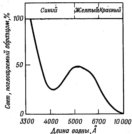
Р и с. 14. Спектр поглощения комплекса [\text{Ti}(\text{H}_2\text{O})_6]^{3+} . Растворы [\text{Ti}(\text{H}_2\text{O})_6]^{3+} окрашены в красно-фиолетовый цвет, так как они поглощают желтые лучи, а пропускают синие и красные.
