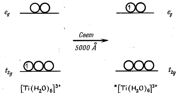
Р и с. 15. d-d -Электронный переход, обуславливающий фиолетовую окраску [\text{Ti}(\text{H}_2\text{O})_6]^{3+} .
