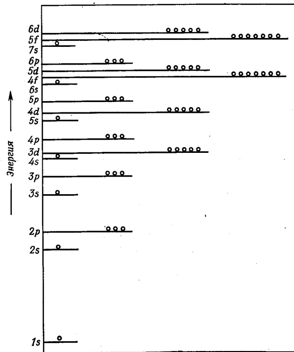
Рис. 1. Схема энергетических уровней орбит легкого атома. На схеме точно указаны относительные значения величин энергии уровней, а абсолютные значения искажены.
