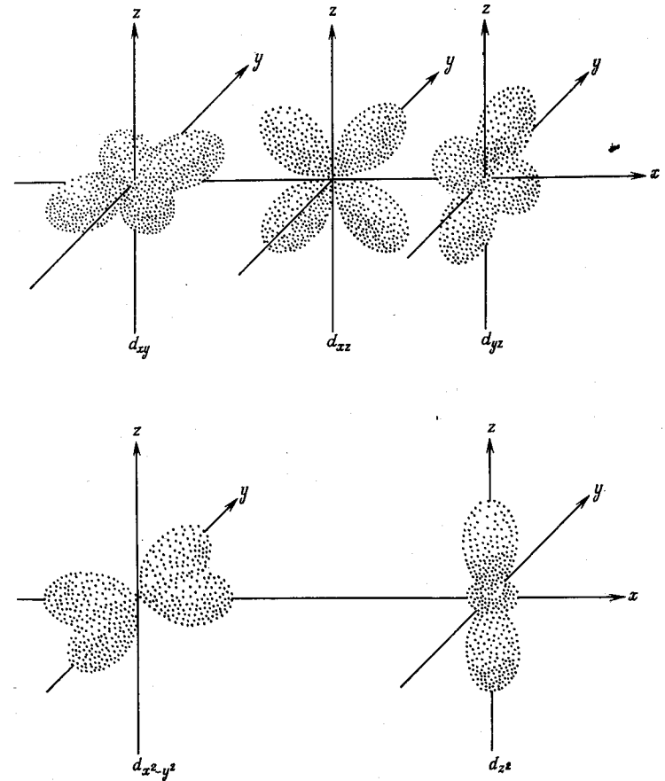
Р и с. 6. Пространственные конфигурации d-орбит.
