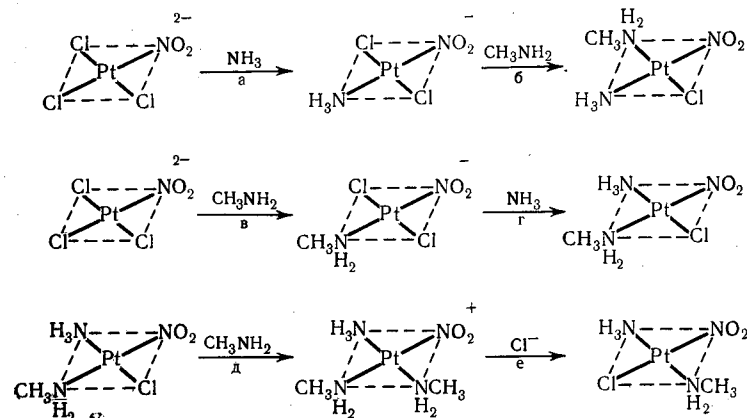
Р и с. 25. Схема приготовления трех изомеров [\text{Pt}(\text{CH}_3\text{NH}_2)(\text{NH}_3)(\text{NO}_2)\text{Cl}] .
